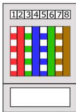
Jedna strana kabelu
