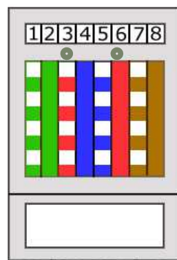
Druhá strana kabelu
